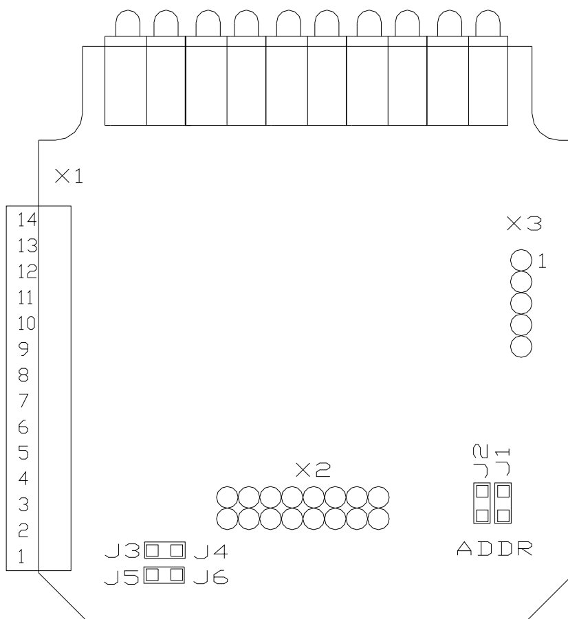
Схема расположения перемычек на плате
