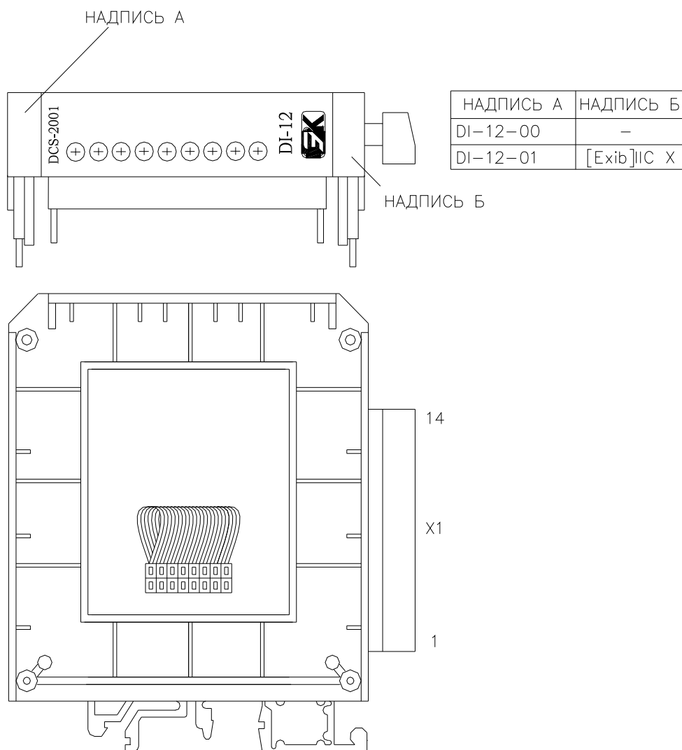
Внешний вид модуля
