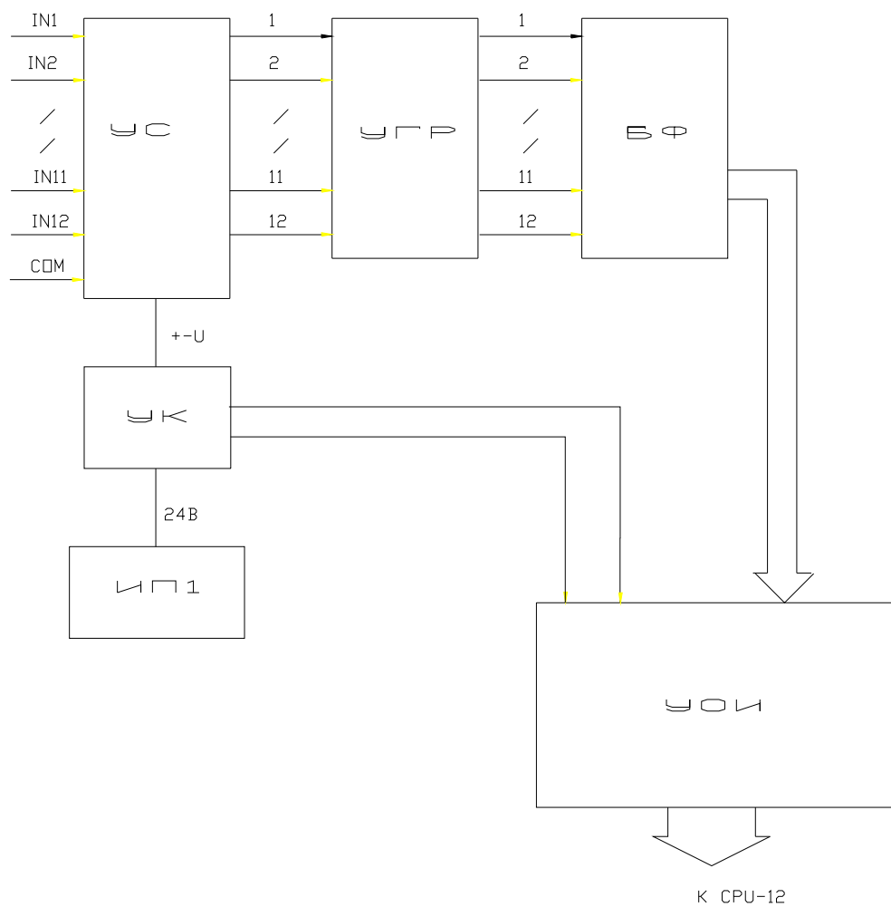
Структурная схема модуля
