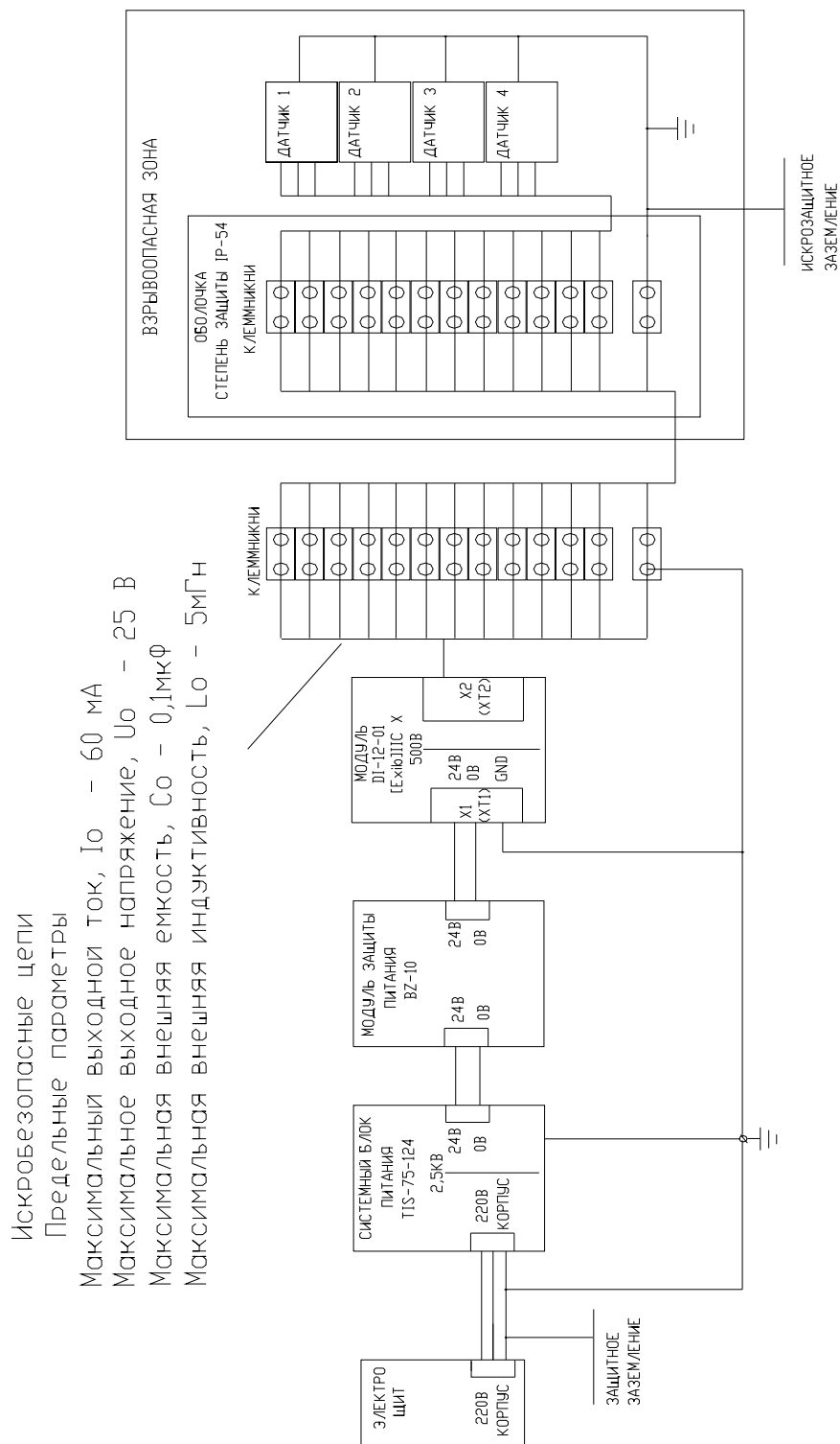
ОБЩАЯ СХЕМА ОБЕСПЕЧЕНИЯ ВЗРЫВОЗАЩИЩЕННОСТИ СИСТЕМЫ. ВИД ВЗРЫВОЗАЩИТЫ МОДУЛЯ GEхЮIIIC X
