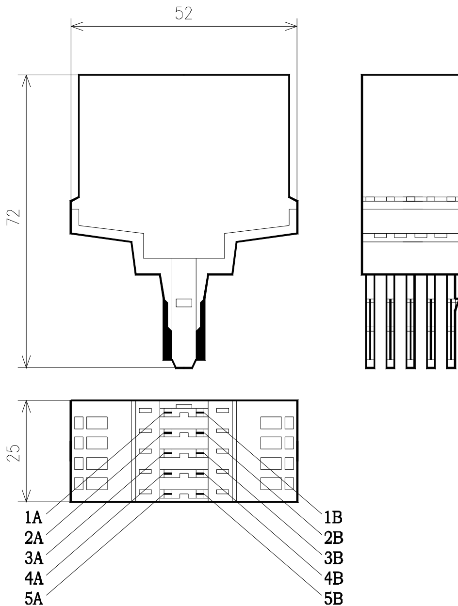
Внешний вид и расположение контактов блока грозозащиты BZ-22
