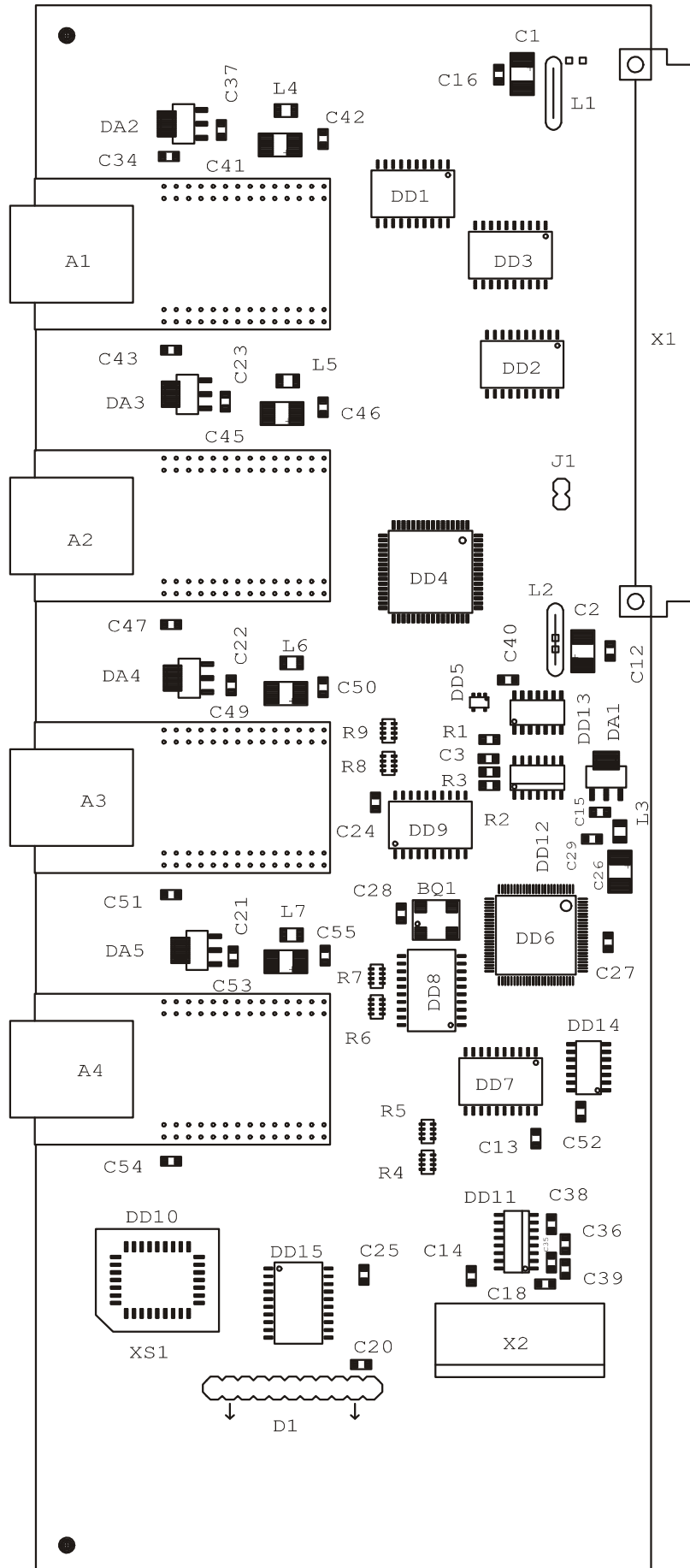
Внешний вид модуля
