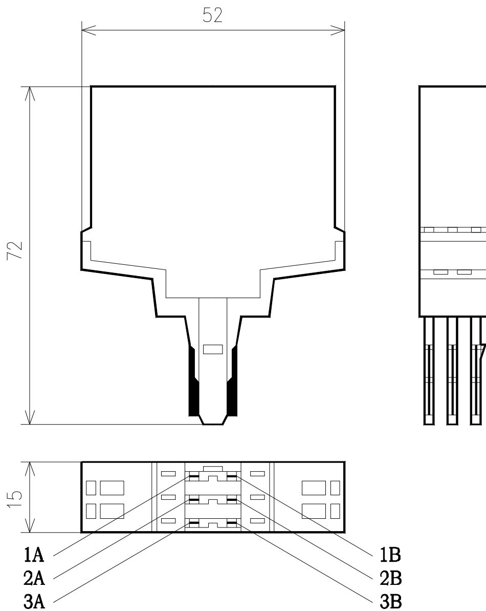
Внешний вид и расположение контактов блока грозозащиты BZ-24
