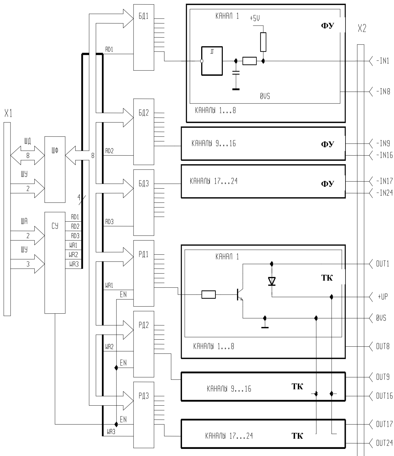
Структурная схема модуля дискретного ввода/вывода DIO-04
