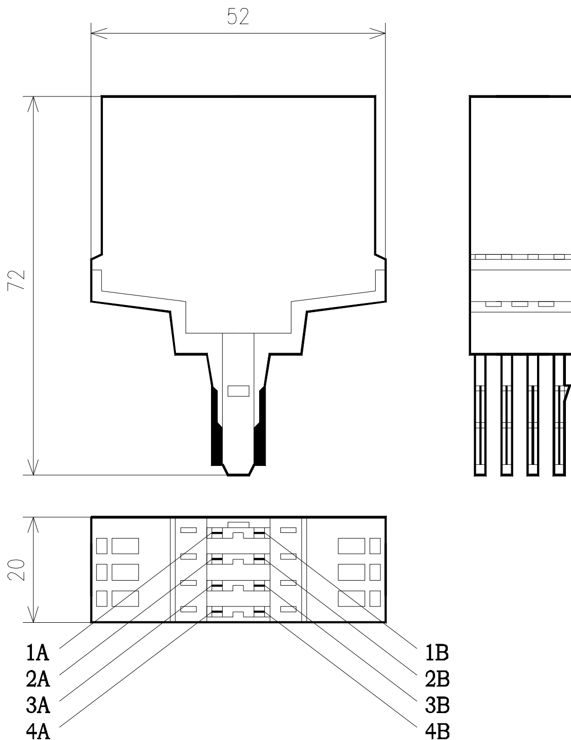
Внешний вид и расположение контактов блока грозозащиты ВZ-25
