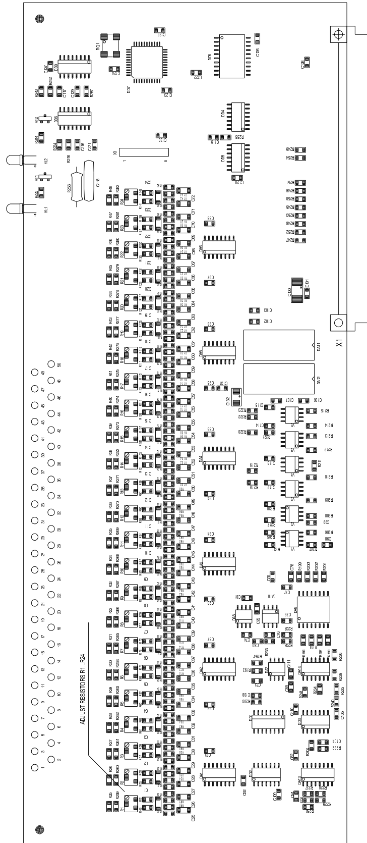
Расположение элементов на плате модуля
