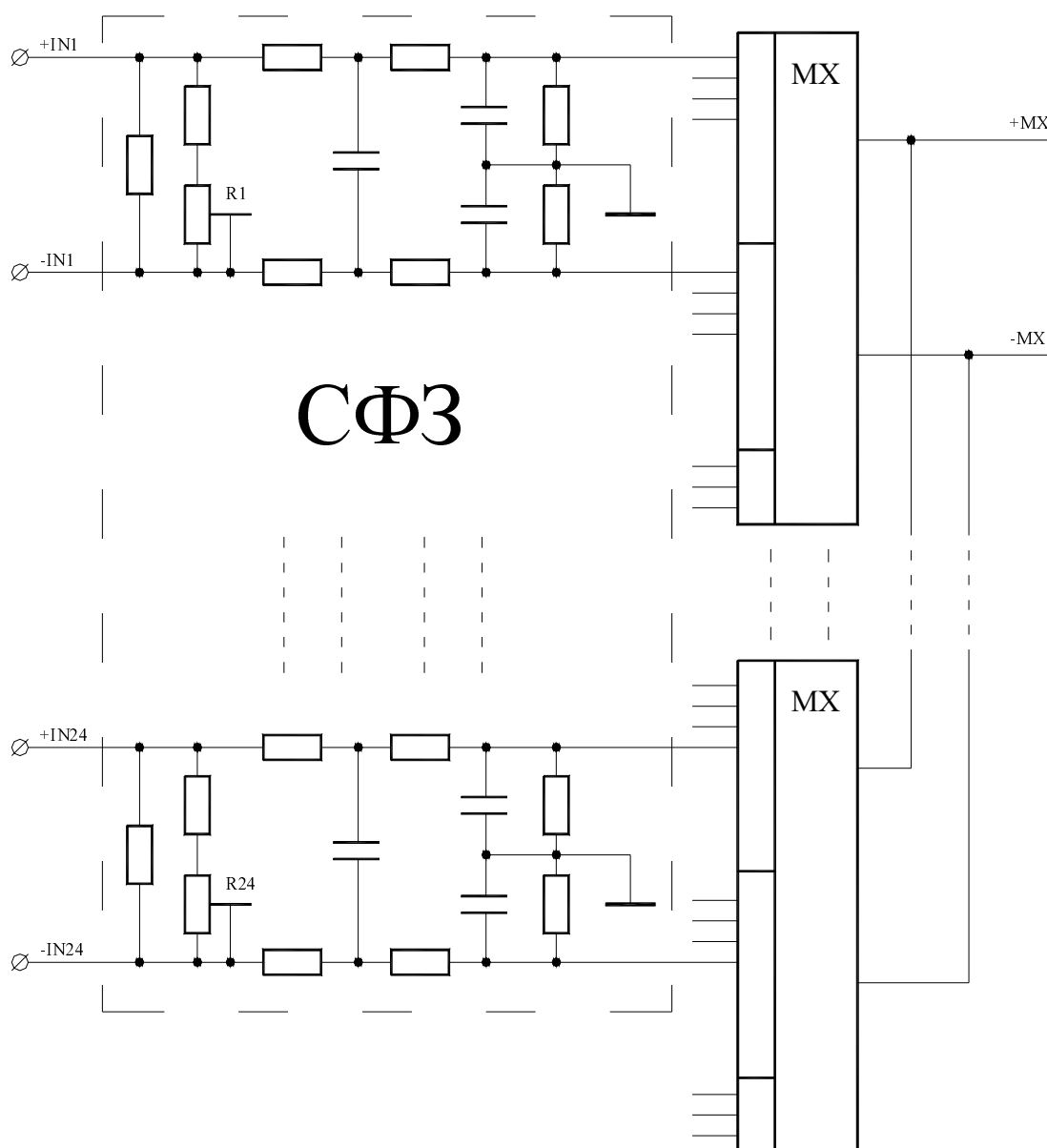
Принципиальная схема входной части модуля
