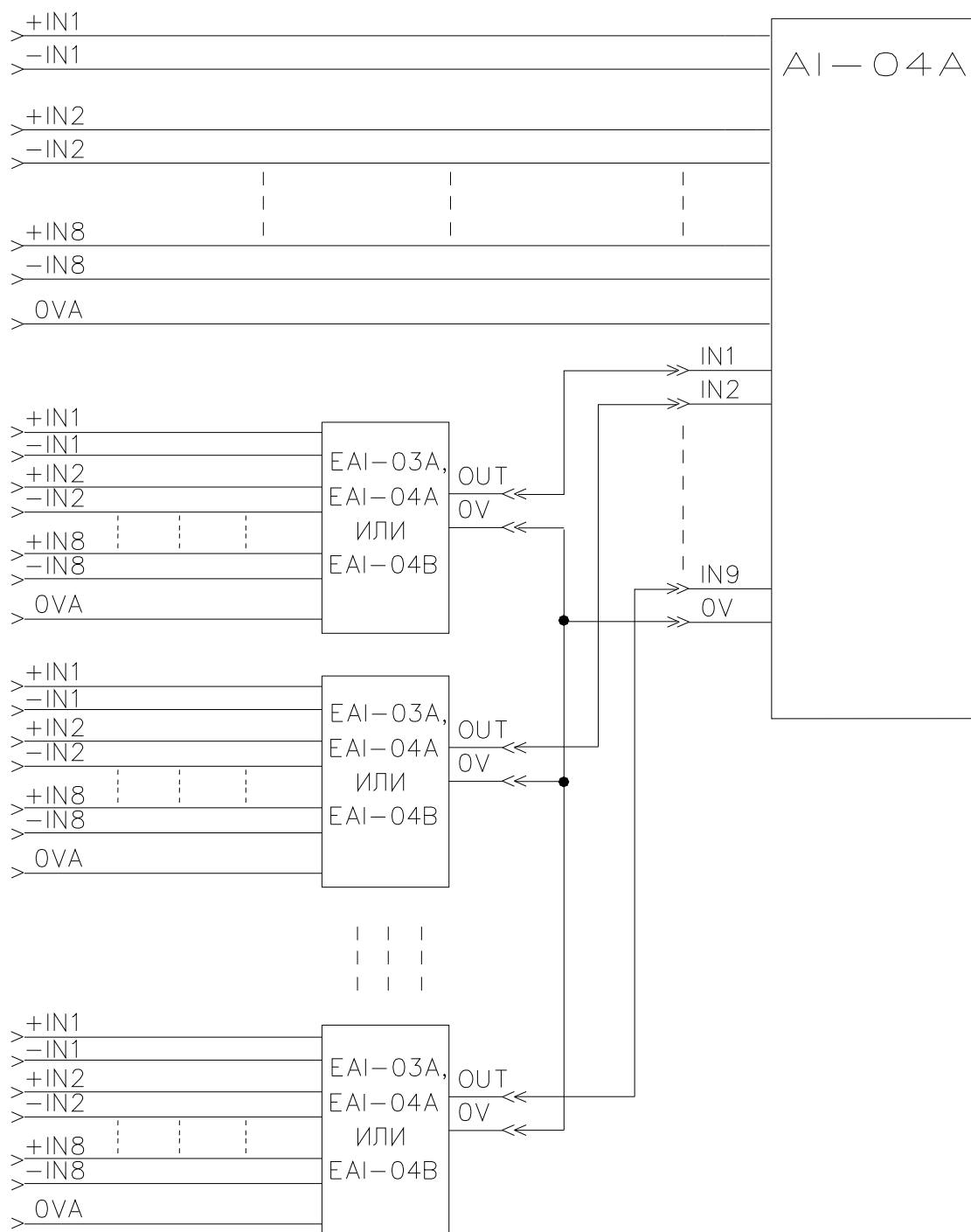
ПРИМЕР ПОДКЛЮЧЕНИЯ МОДУЛЕЙ РАСШИРЕНИЯ
