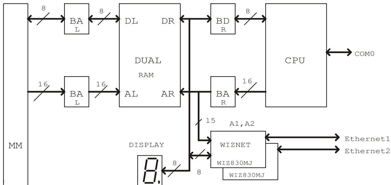
Структурная схема модуля
