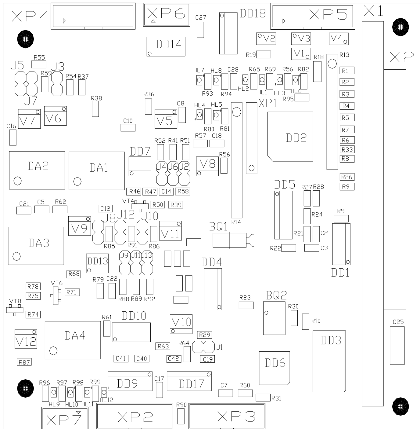
Внешний вид модуля со стороны компонентов
